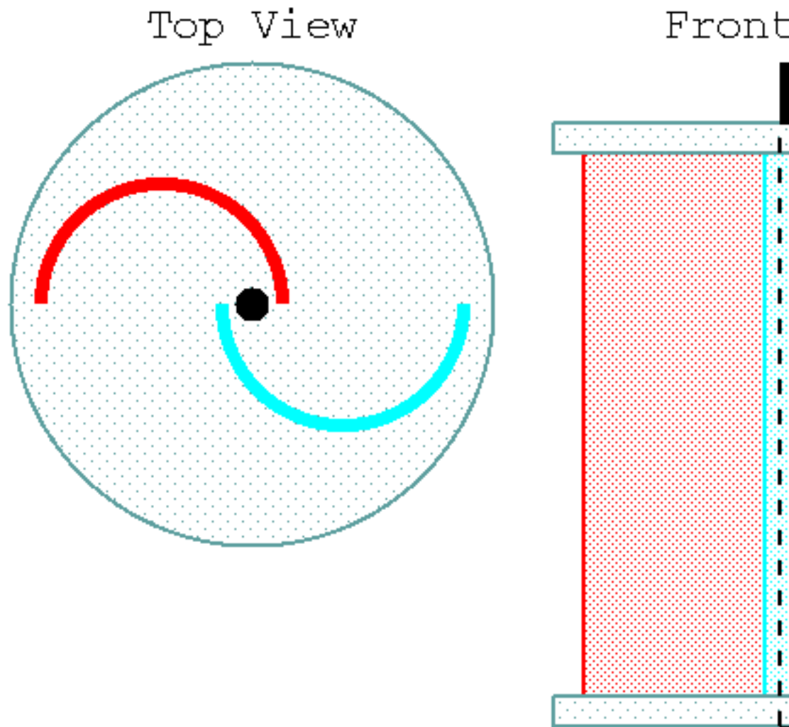
Savonius Rotor
